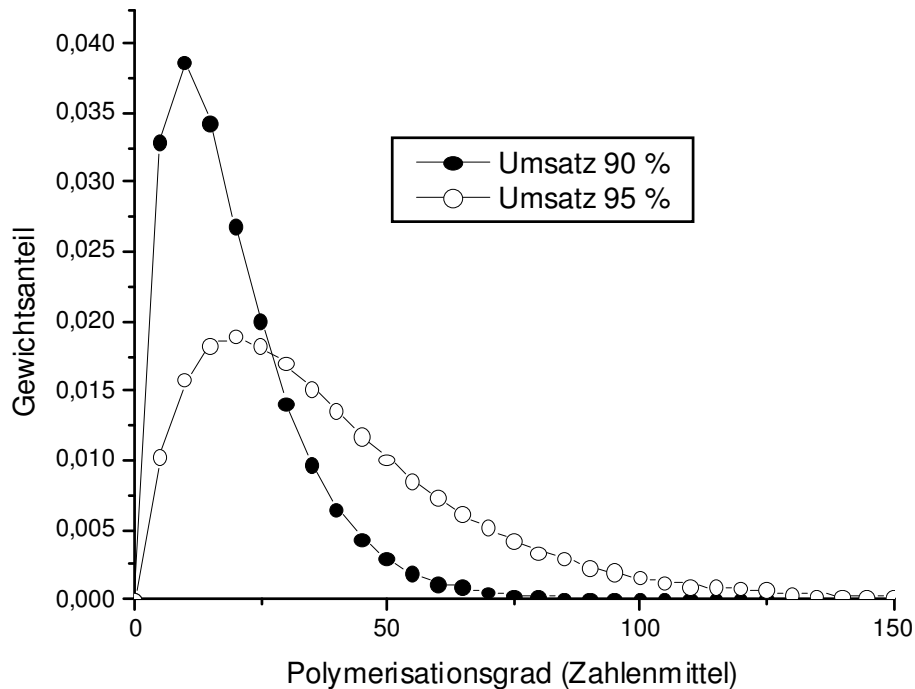
Abbildung 3.5: Molekularmassenverteilung für eine Stufenreaktion in Abhängigkeit vom Polymerisationsgrad für verschiedene Umsatzgrade.
