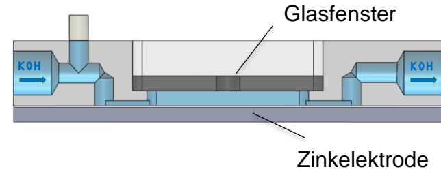
Abb.1: Messzelle
